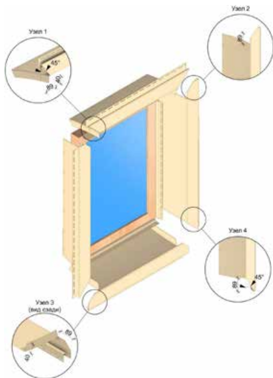
Рис. 8 Обрамление оконного проёма при помощи околооконного профиля 89 мм/ 30 мм.
