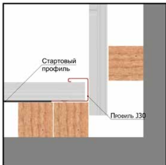
Рис. 10 Отделка с помощью профиля J30.
