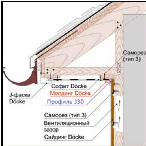
Рис. 17 Примыкание сайдинга Döcke LUX под камень к карнизному свесу.
