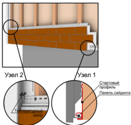
Рис. 12 Монтаж первой панели сайдинга
