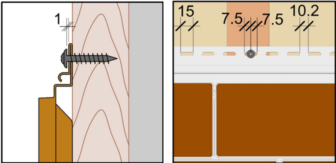
Рис. 2 Схема фиксации сайдинга Döcke LUX под камень
