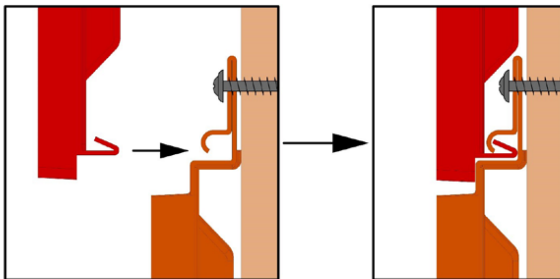
Рис. 16 Соединение панелей верхнего и нижнего ряда между собой
