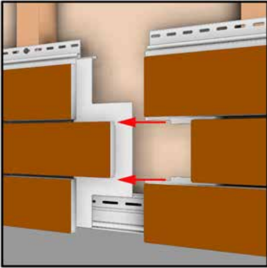
Рис. 13 Монтаж последующих панелей первого ряда сайдинг
