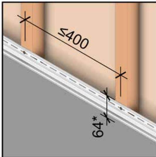
Рис. 4 Установка стартового профиля
