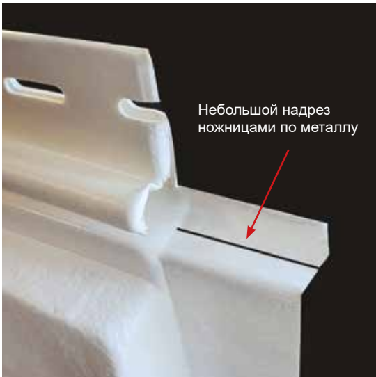
Рис. 14 Усиление жёсткости вертикального соединения панелей (необходимо выполнять при отдалении стойки обрешётки на расстоянии более 100 мм)
